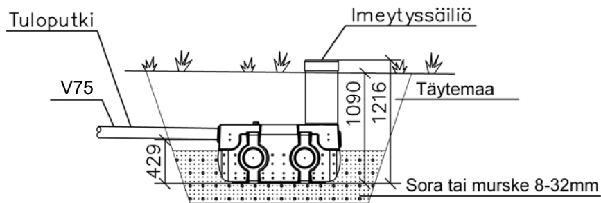
Imeytyssäiliö, reijitetty 0,3 m 3
